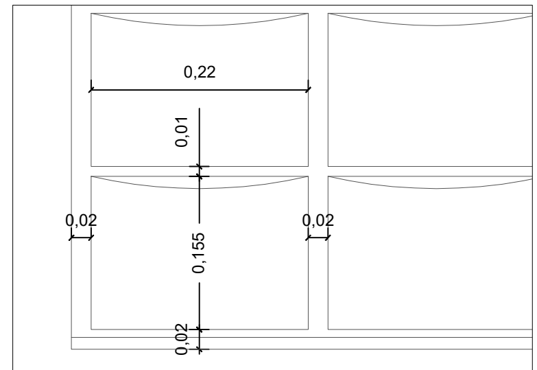
detalle B
