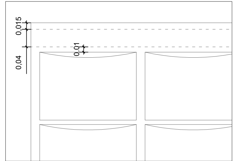
detalle A
